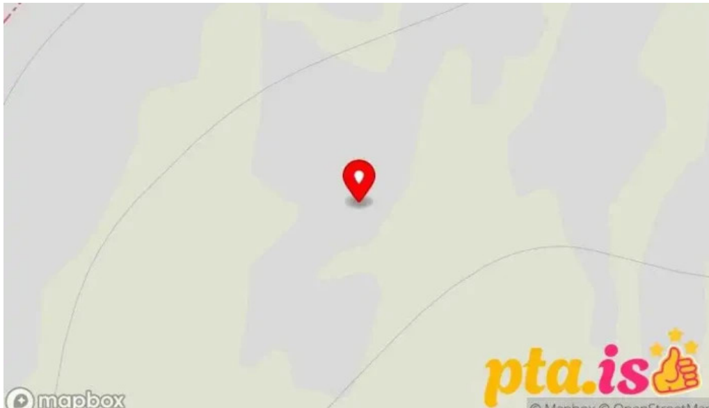
Glaesithufa iceland
