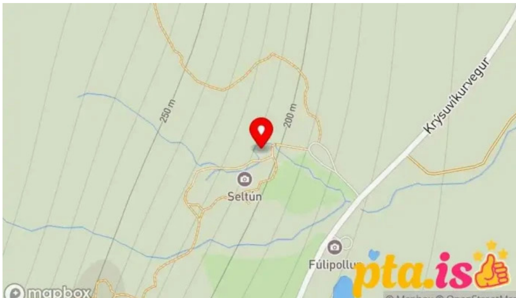
Seltun geothermal area Kort
