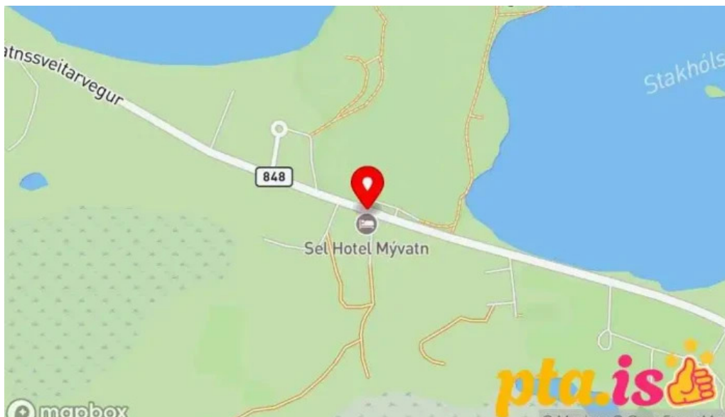
Skutustadagrig pseudo craters Kort
